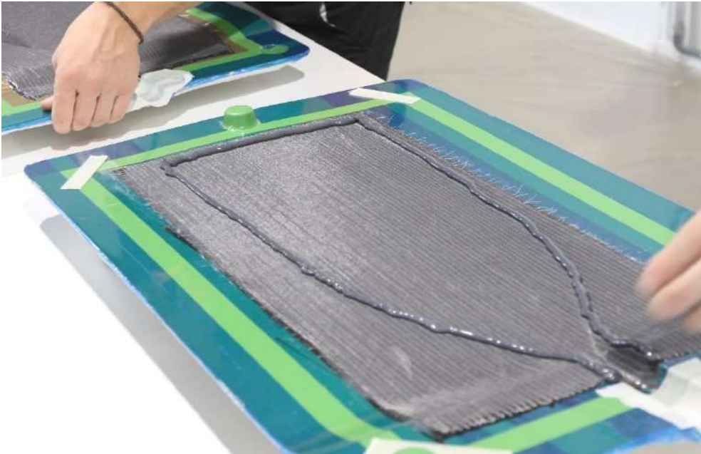
Aplicación de adhesivo de metacrilato Crestabond M1-20 sobre remo fabricado con resina epoxi y tejidos de carbono
